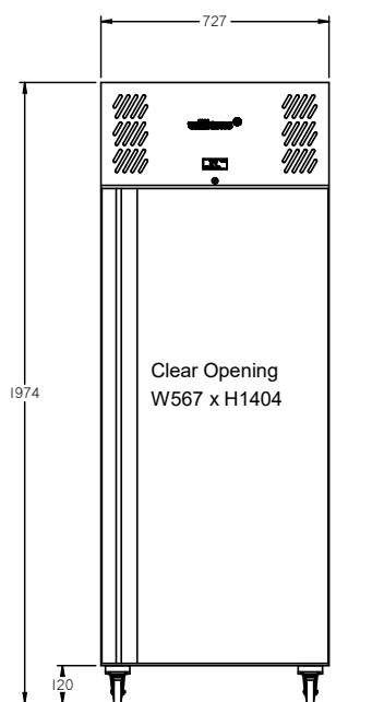
ELEVATION
