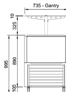
End Elevation
