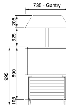
End Elevation
